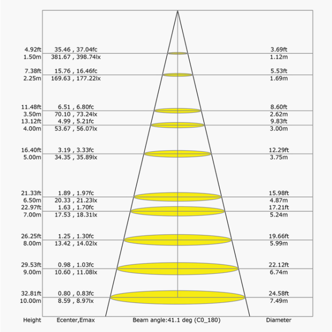
Diagrama cónico 45°. Beam cone diagram 45°
