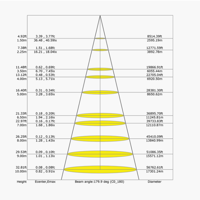
Diagrama cónico 15°. Beam cone diagram 15°
